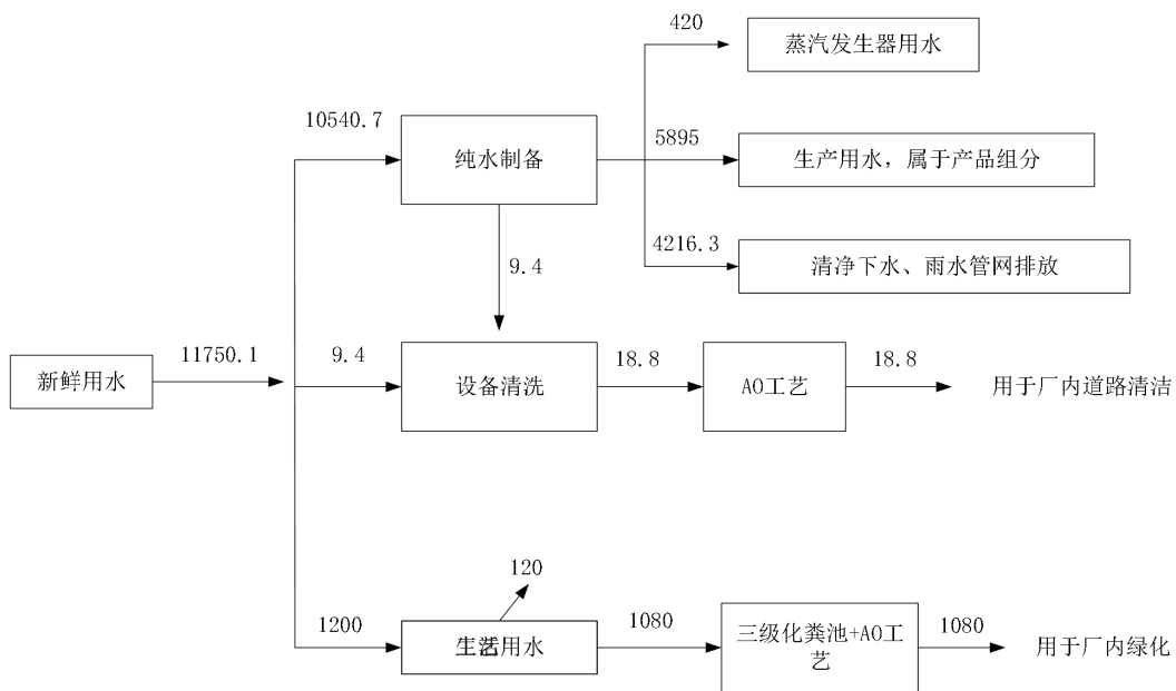
图 2-1 项目用水平衡图单位 t/a
