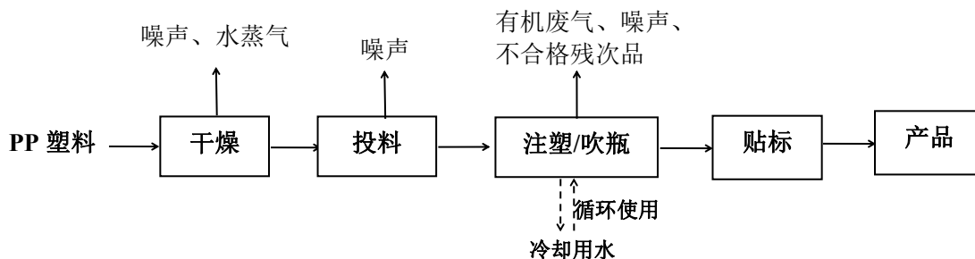
图2-2 项目包装瓶生产线工艺流程图
