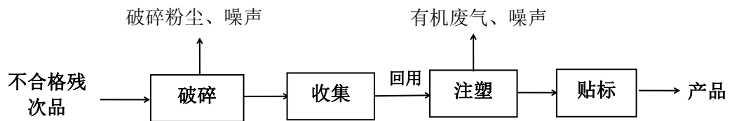
图2-3 项目残次品回用生产线工艺流程图
